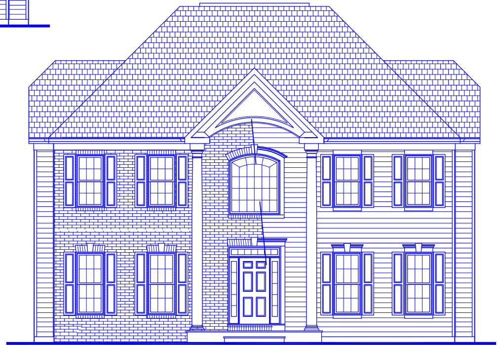
ELEV. B
